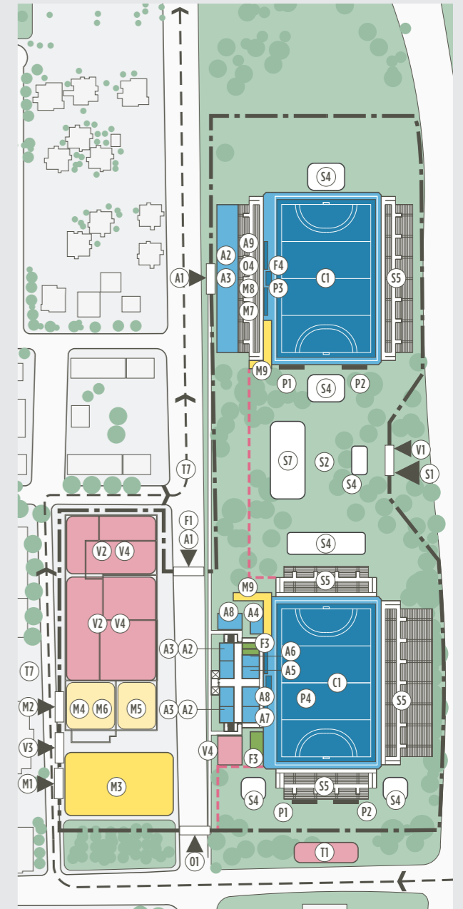
Plan de masse détaillé, niveau 1 Detailed block plan, level 1
