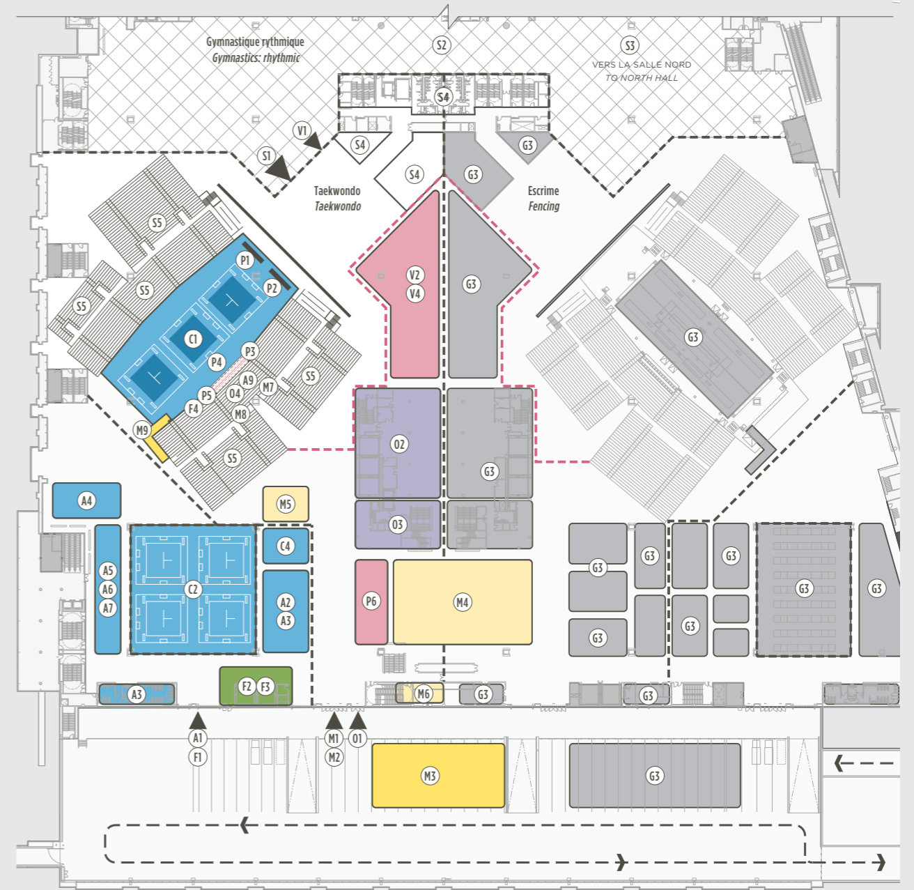
Plan de masse détaillé : hall ouest, niveau 3 Detailed block plan: West Hall, level 3
