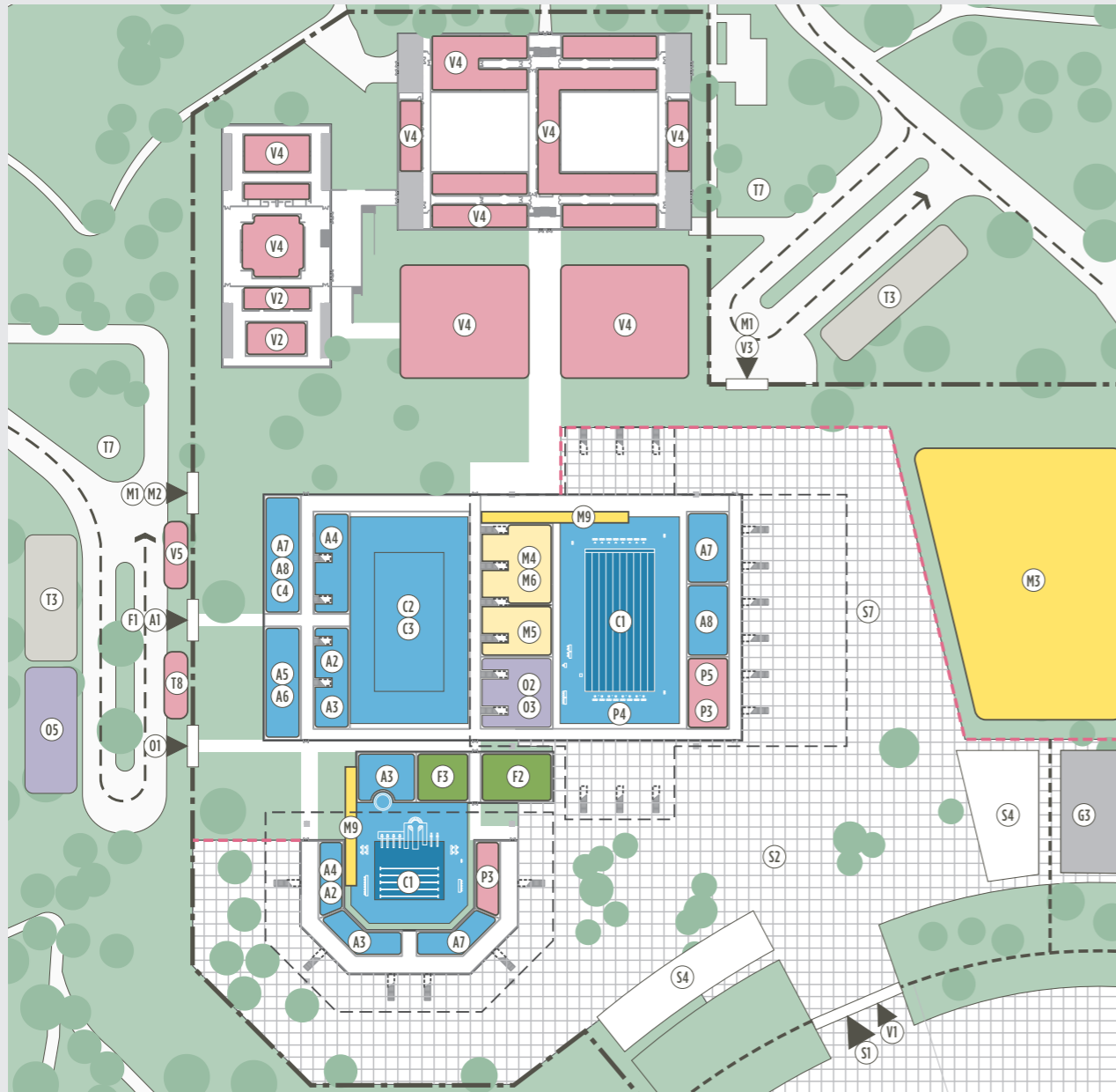
Plan de masse détaillé, niveau 1 Detailed block plan, level 1
