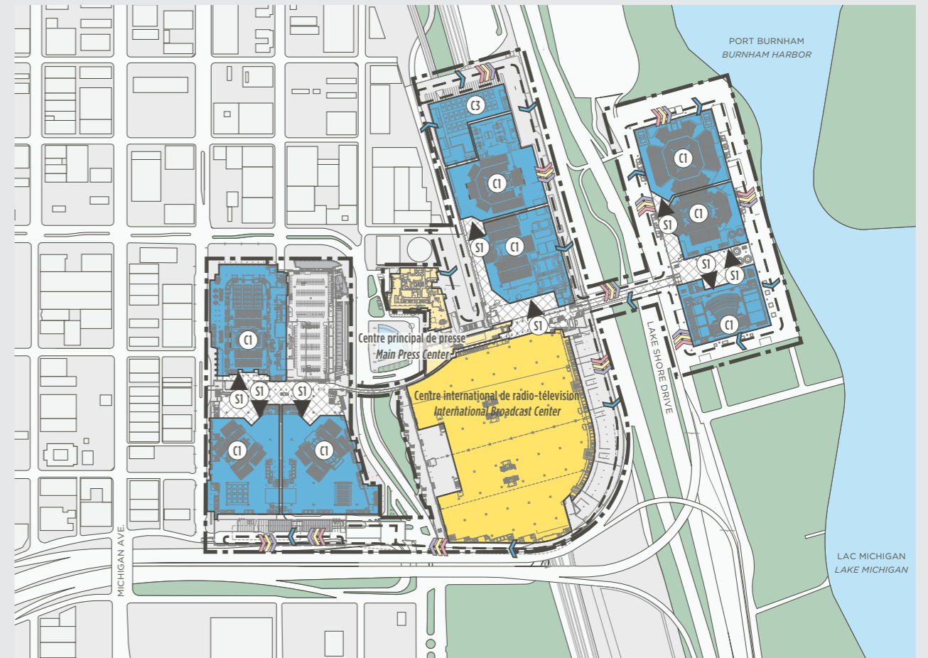
Plan de masse du secteur : niveau 3 Precinct block plan: level 3
