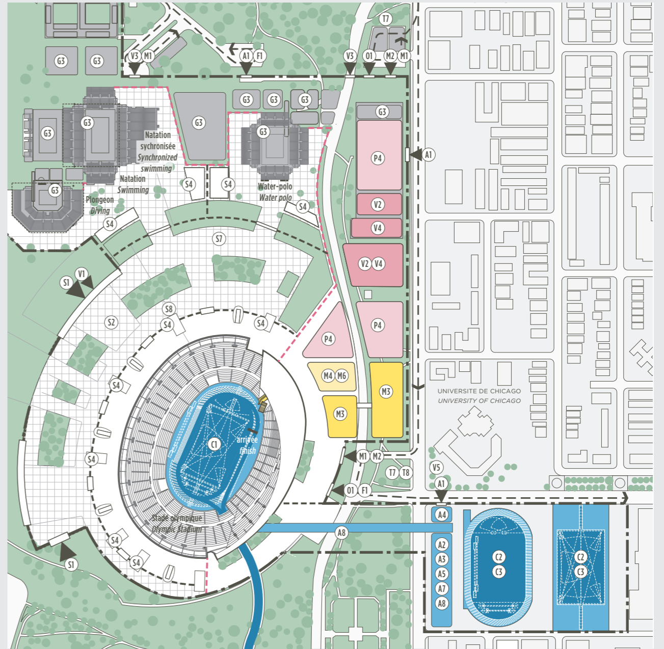
Plan de masse détaillé Detailed block plan
