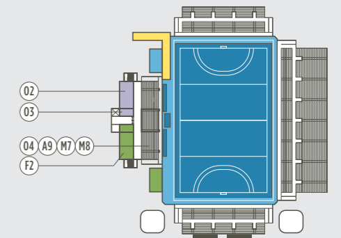
Plan de masse détaillé, niveau 2 Detailed block plan, level 2
