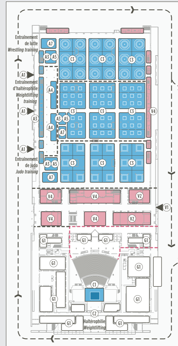
Plan de masse détaillé : hall est, niveau 2 Detailed block plan: East Hall, level 2
