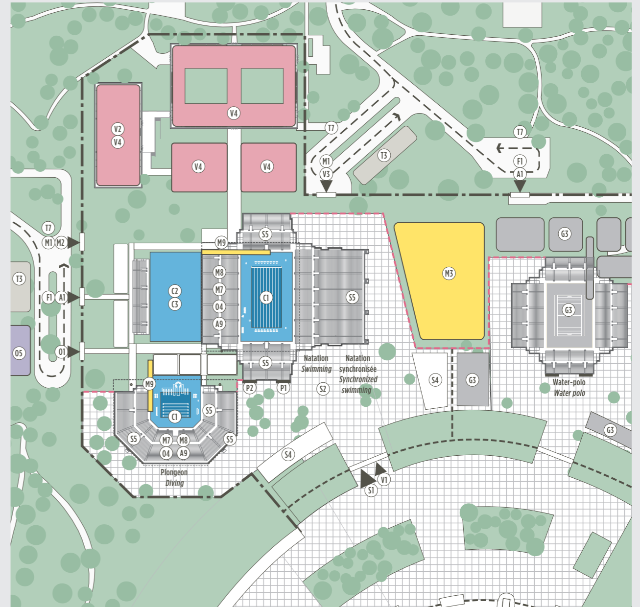
Plan de masse détaillé, niveau 2 Detailed block plan, level 2
