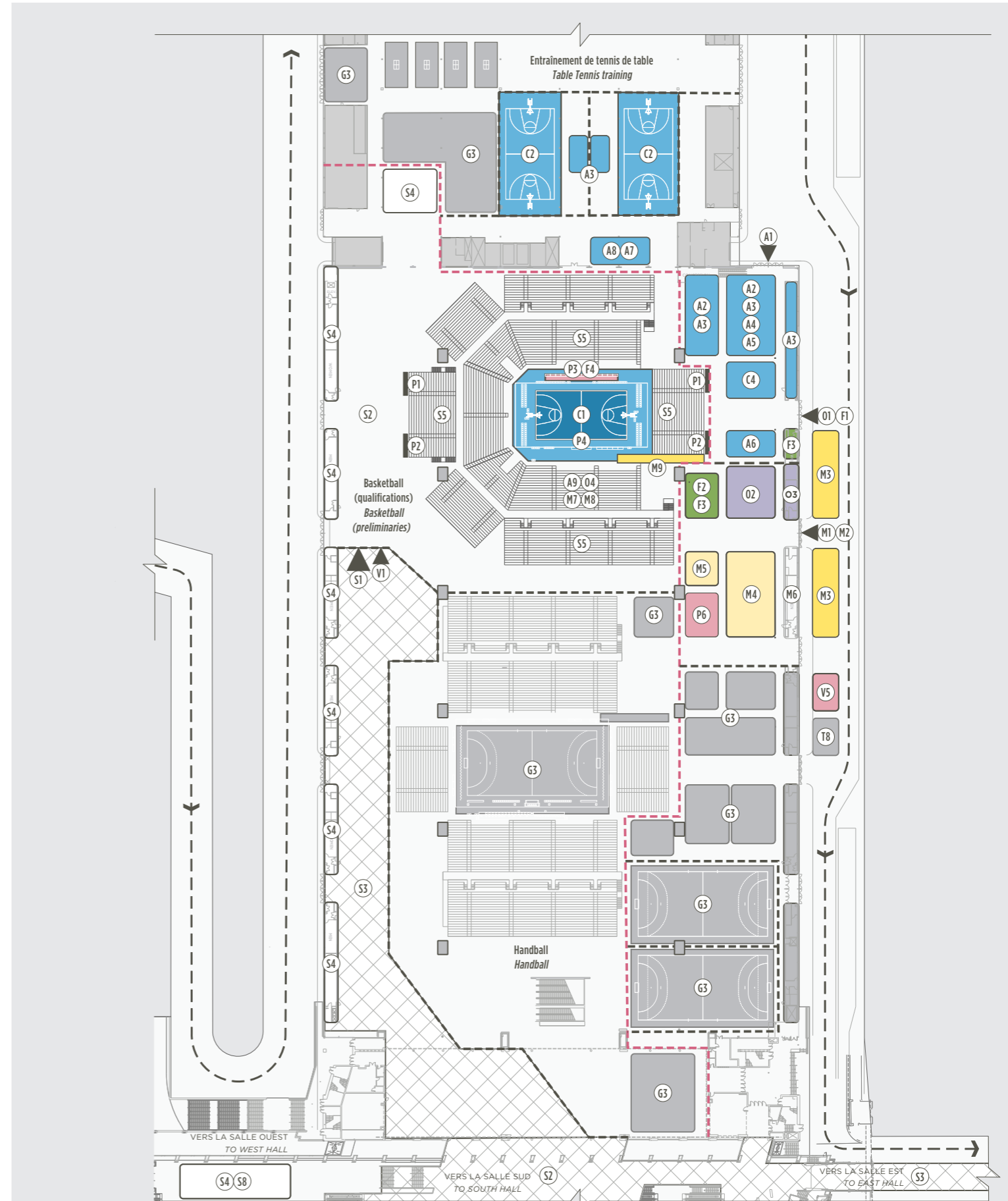
Plan de masse détaillé : hall nord, niveau 3 Detailed block plan: North Hall, level 3
