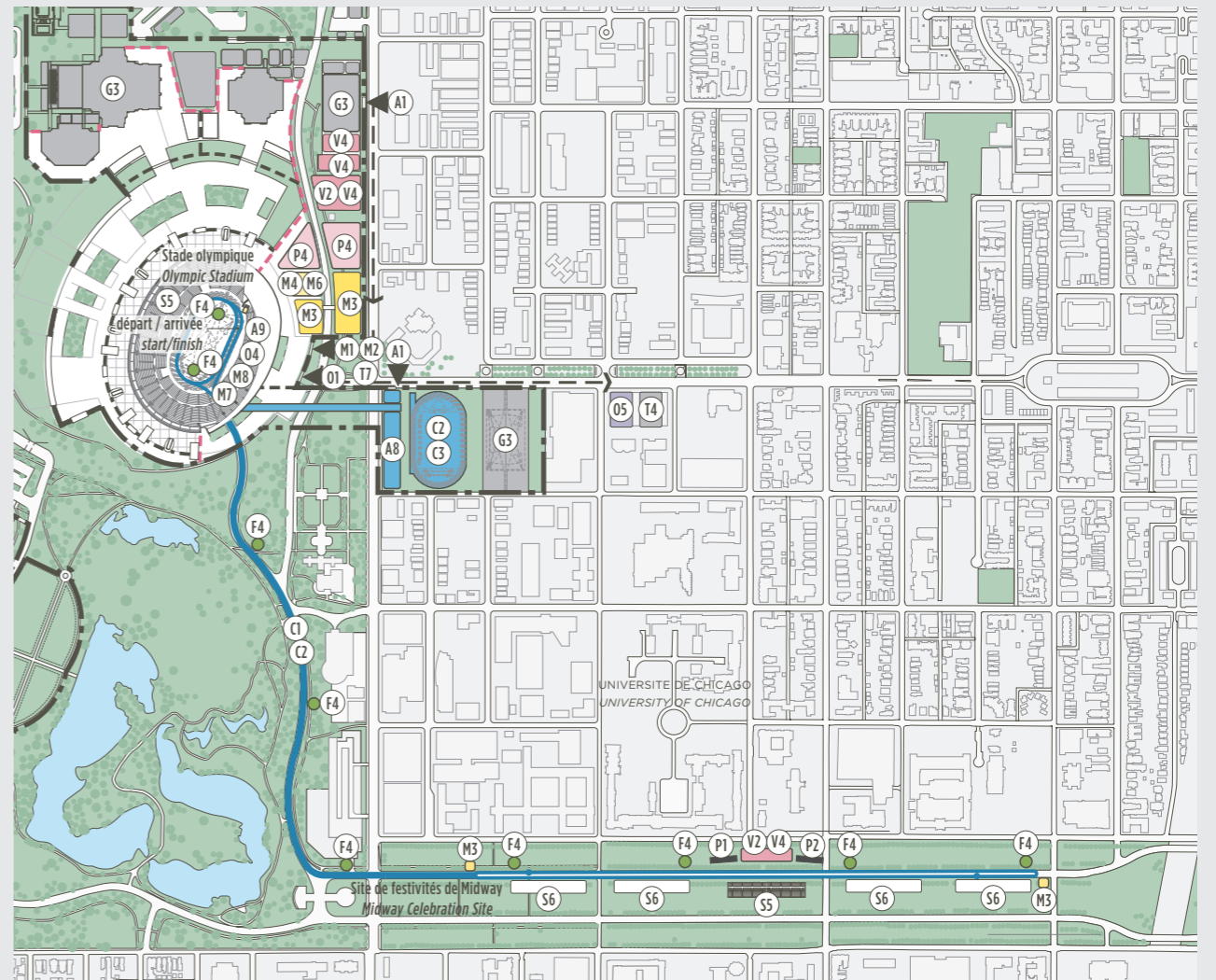
Plan de masse détaillé, marche Detailed block plan, race walk
