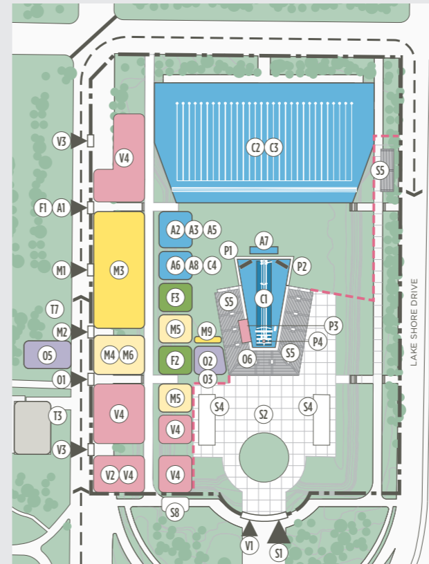
Plan de masse détaillé Detailed block plan
