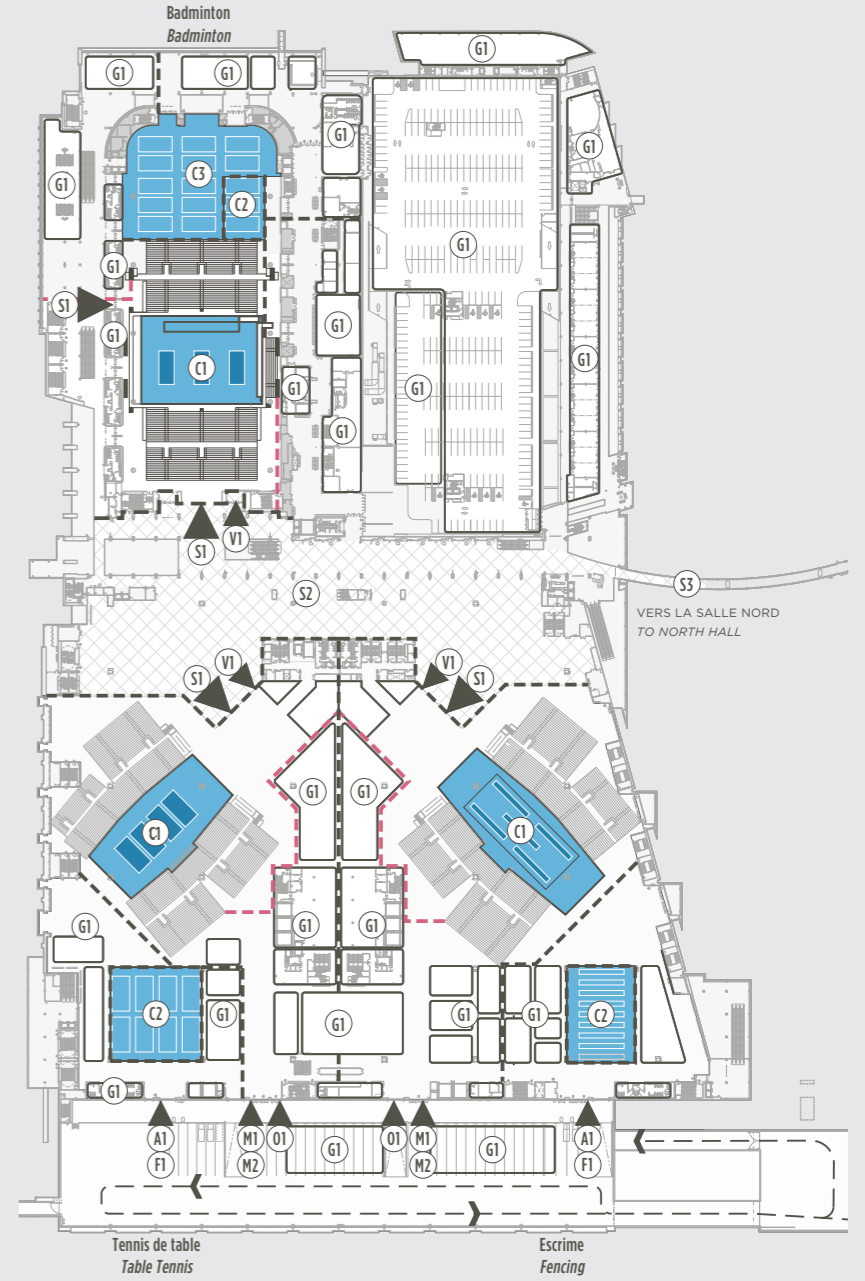
Plan de masse du site : hall ouest, niveau 3 Venue block plan: West Hall, level 3
